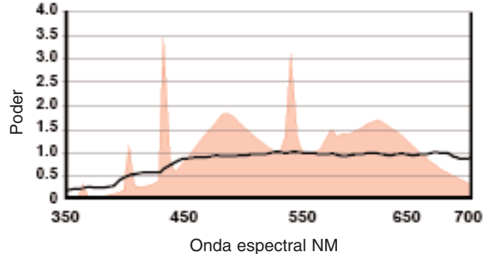
Distribución espectral Lámpara de D50 comercialmente disponible
