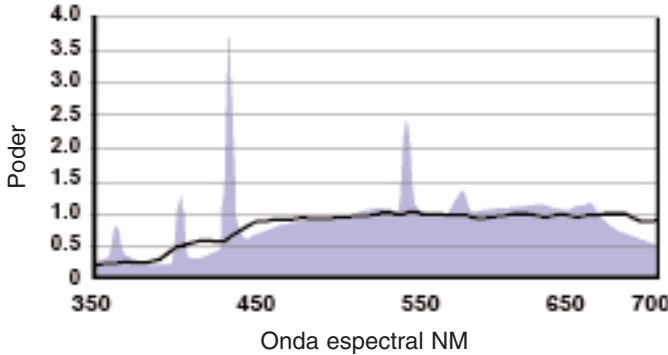
Distribución espectral Lámpara Graphiclite 100 de D50
